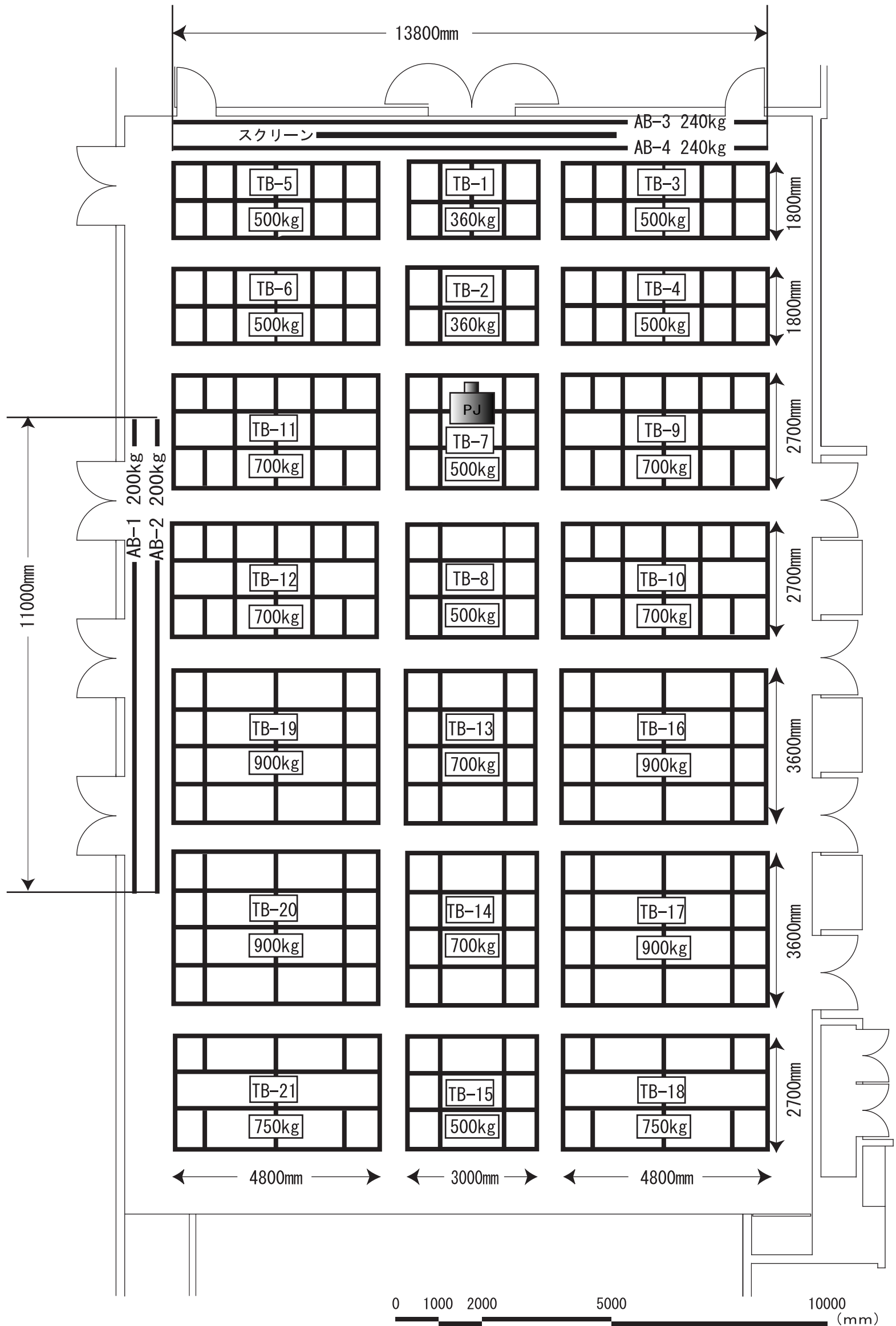
トラス・バトン詳細図 (トラス直径42.7mm)
